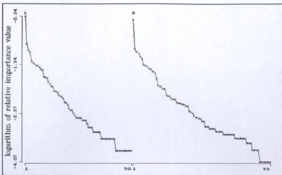
نمودار (۱-۲) پلات دسته - فراوانی برای دو منطقه بر اساس داده های مربوط به پوشش تاجی
