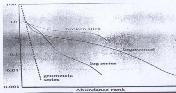
شکل (۱-۱): نمایش مدل های فراوانی گونه ای
