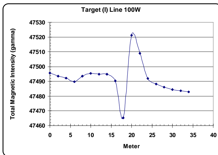
شکل ۱۴- پروفیل مغناطیس‌سنجی 100W از غرب منطقه اکتشافی (۱). جهت حرکت شمال - جنوب
