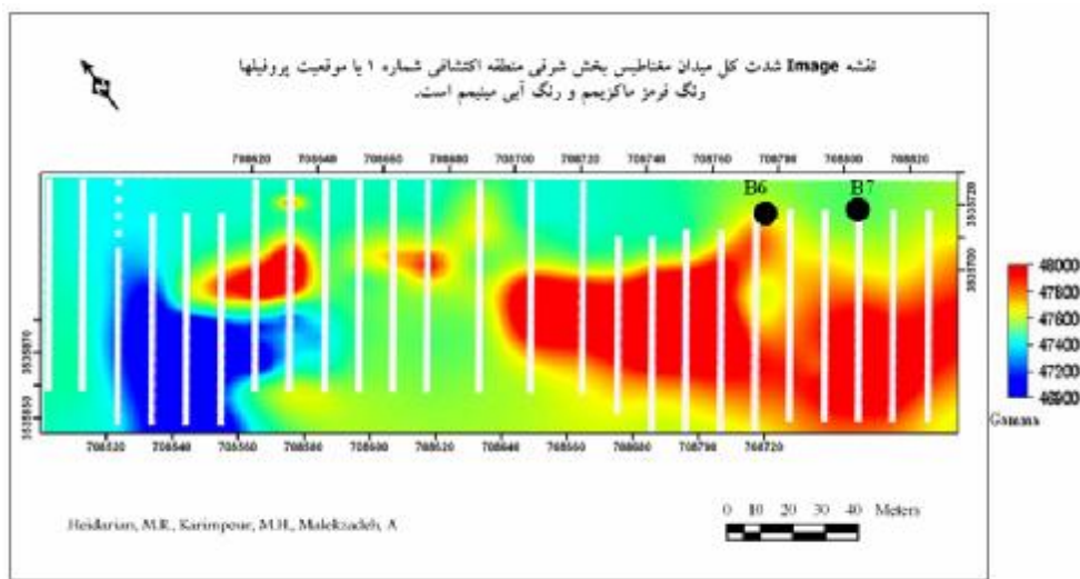
نقشه ۹- نقشه Image شدت کل میدان مغناطیسی شرق منطقه اکتشافی (۱) همراه با موقعیت پروفیل‌های ژئوفیزیکی
