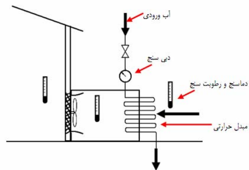
شکل ۳- طرح شماتیک سرمایه‌شمر مرکب
