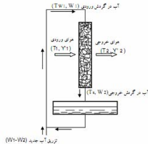
شکل 1- اصول کار کولرهای آبی (ایده آل آدیباتیک)
