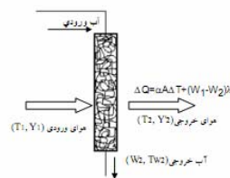
شکل 2- کولر آبی غیر آدیاباتیکی
