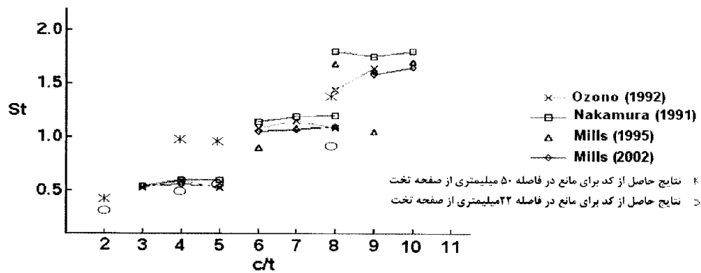
شکل ۶- تغییرات عدد اشتروهال با نسبت c/t
