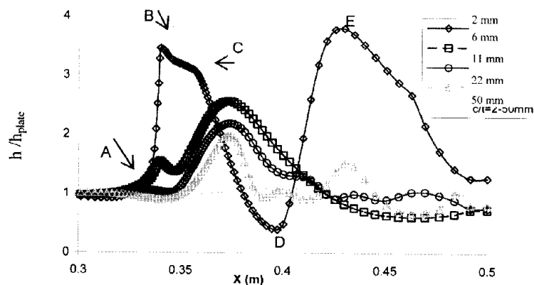
شکل ۱۰- تغییرات ضریب انتقال گرما روی صفحه تخت تحت تاثیر مانع با نسبت ابعادی c/t = 2 . هر منحنی مربوط به یکی از فاصله‌های d = [2, 6, 11, 22, 50] mm از صفحه تخت است. هر دو مقدار h و h_{plate} به صورت موضعی و مربوط به یک نقطه از صفحه هستند.
