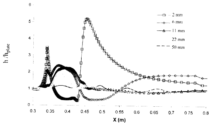
شکل ۱۲- تغییرات ضریب انتقال گرما روی صفحه تخت، تحت تاثیر فاصله مانع از صفحه تخت ( c/t=8 ) هر دو مقدار h و h_{plate} به صورت موضعی و مربوط به یک نقطه از صفحه هستند.
