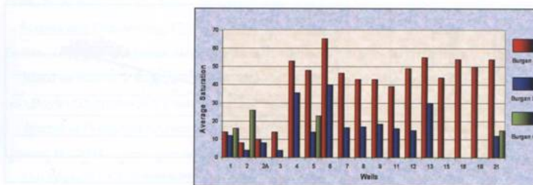
شکل ۱۵- نمودار میانگین اشباع شدگی محاسبه شده برای افق‌های A, B, C سازند بورگان در چاه‌های مختلف
