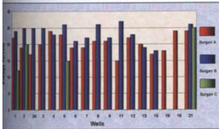
شکل ۱۰- نمودار میانگین تخلخل محاسبه شده برای افشای A, B, C بورگان در چاه‌های مختلف
