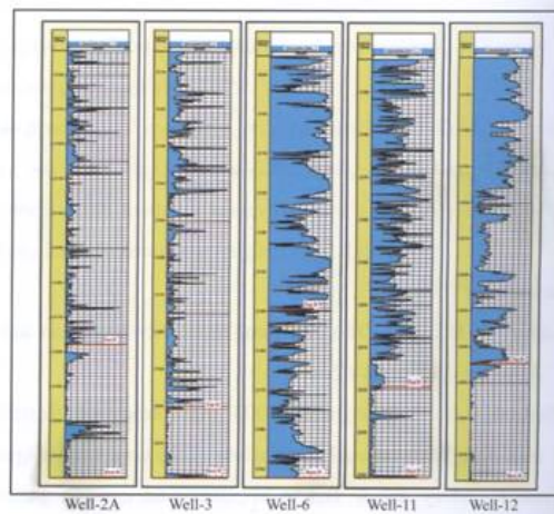
شکل ۱۸- نگاره‌های اشباع شدگی در چاه‌های مختلف میدان مورد مطالعه
