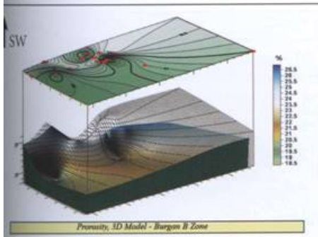
شکل ۱۲- مدل سه بعدی نحوه توزیع تخلخل در زون B سازند بورگان در کل میدان
