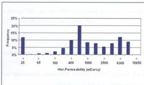
شکل ۱۹- فراوانی تراوایی به دست آمده از داده‌های مغزه در زون B سازند بورگان
