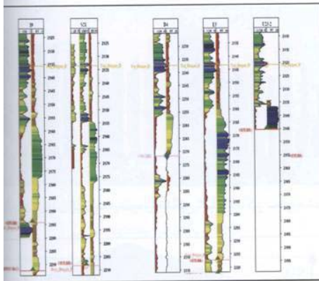
شکل ۲۱- رسم نگارهای مقاومت ویژه کل و حجم شیل در چاه‌های مختلف برای تعیین سطح تماس آب-نفت
