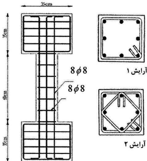
شکل ۱- جزئیات ستون‌های آزمایش شده
