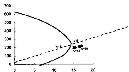
شکل ۳- نمودارهای اندرکنش نیروی محوری و لنگر خمشی و نتایج آزمایش
