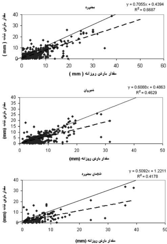
شکل ۲- مقایسه ی مقادیر قرائت شده از باران سنج روزانه و مقادیر بارش ثبت شده در باران سنج های ثابت استان خراسان شمالی. خط ممتد خط تطابق آرمانی (شیب ۱:۱) و خط منقطع خط رگرسیون می باشد. در کلیه ی حالات p -مقدار از 0.0001 کوچکتر و سطح اعتماد از 0.9999 بزرگتر است.
