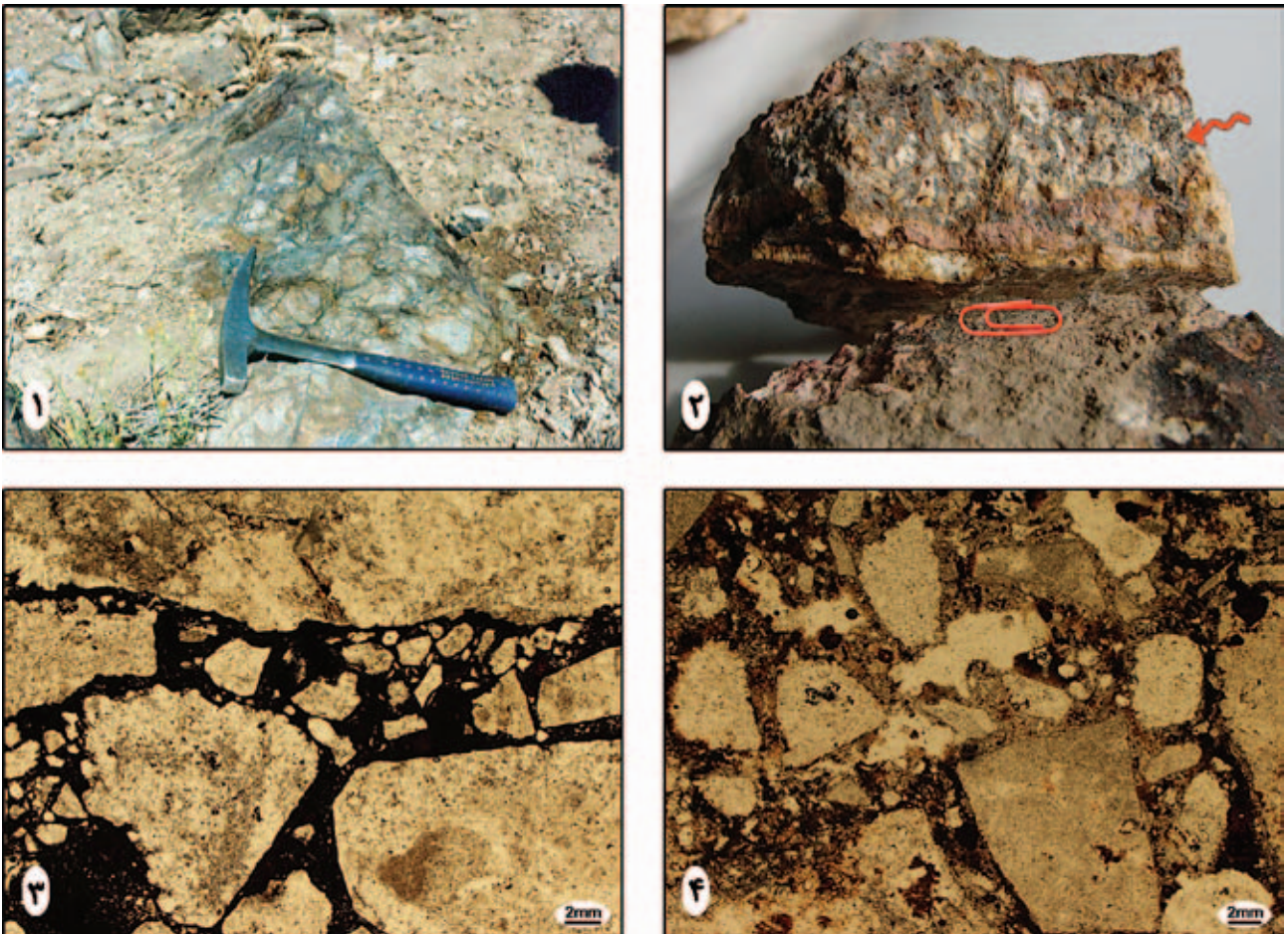
شکل ۹- سیلیس با بافت برشی ۱- در صحرا ۲- در نمونه دستی ۳- مقطع نازک از بافت برشی با سیمان پیریت، مقطع شماره ۲۰، PTN، PPL ۴- برش با قطعات ولکانیکی، مقطع شماره ۳۰، PTN، PPL
