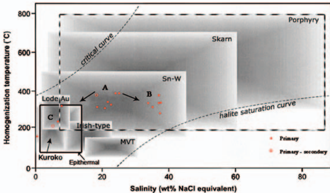
شکل ۱۶- محل قرارگیری سیالات نمونه‌های تنورچه (A, B, C) در نمودار درجه همگن‌سازی در مقابل شوری کانسارهای مختلف (ویلکینسون ۲۰۰۱ با تغییر) [۲۳]، محدوده خط چین مربوط به کانسارهای پورفیری و محدوده مشخص شده با خط ممتد مربوط به کانسارهای اپی ترمال می‌باشد.
