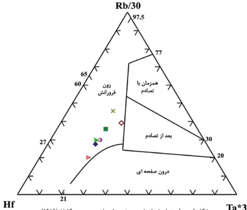
شکل ۶ - موقعیت نمونه‌های نیمه عمیق در نمودار هریس و همکاران (۱۹۸۶)
