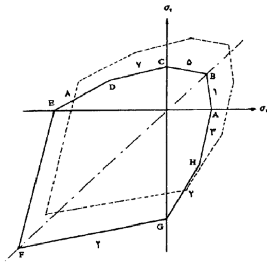
شکل ۱- سطح تسلیم ترسکاگونه نوع چهارم با قانون سخت شوندهگی ترکیبی
