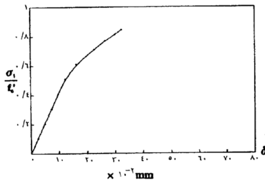
شکل ۱۰- نمودار بار - تغییر مکان نمونه بتنی کاپفر
