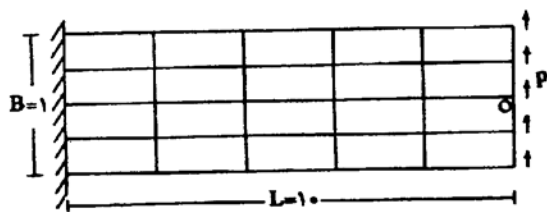
شکل ۲- نمونه خمشی تیر یکسرگیردار
