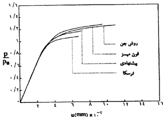
شکل ۳- نمودار بار تغییر مکان نمونه خمشی تیر یکسرگیردار
