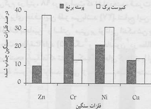
شکل ۳- درصد جذب فلزات سنگین توسط پوسته برنج و کمپوست برگ
