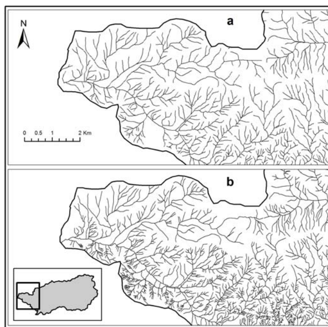
شکل شماره (۵): شبکه‌ی آب‌های مستخرج از نقشه‌های توپوگرافی (a) و عکس‌ها و تصویرهای ماهواره‌ای (b)
