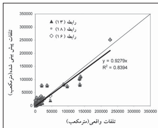
شکل ۵- بررسی روابط (۱۳)، (۱۸) و (۱۶) در یک کیلومتر دهم بازه
