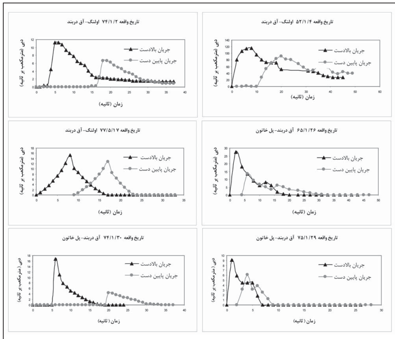
شکل ۲- نمونه هایی از هیدروگراف های سیل مشاهداتی
