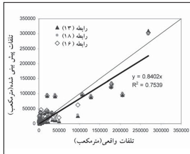
شکل ۳- بررسی روابط (۱۳)، (۱۸) و (۱۶) در یک کیلومتر اول بازه (خط برازش داده شده مربوط به رابطه (۱۶) است)
