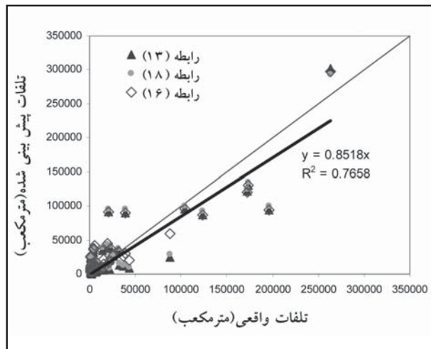
شکل ۴- بررسی روابط (۱۳)، (۱۸) و (۱۶) در یک کیلومتر دوم بازه
