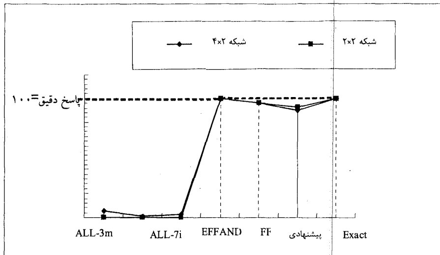
شکل ۷. نتیجه‌های تحلیل عددی نمونه (۹-۳)
