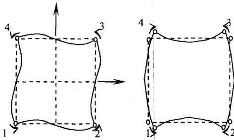
شکل ۲. حالت‌های نادرست در جزء چهارپهلوی غشایی [۱۲]
