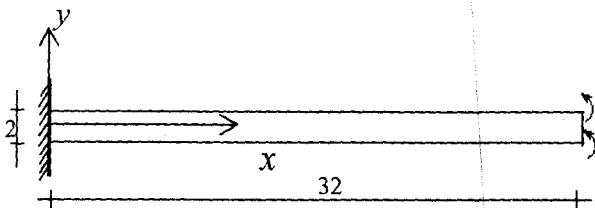
شکل ۶. تیر طره‌ای با لنگر
