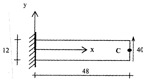
شکل ۵. تیر طره‌ای با نیروی برشی در انتها جدول ۴. تغییر مکان سر تیر طره‌ای با برش
