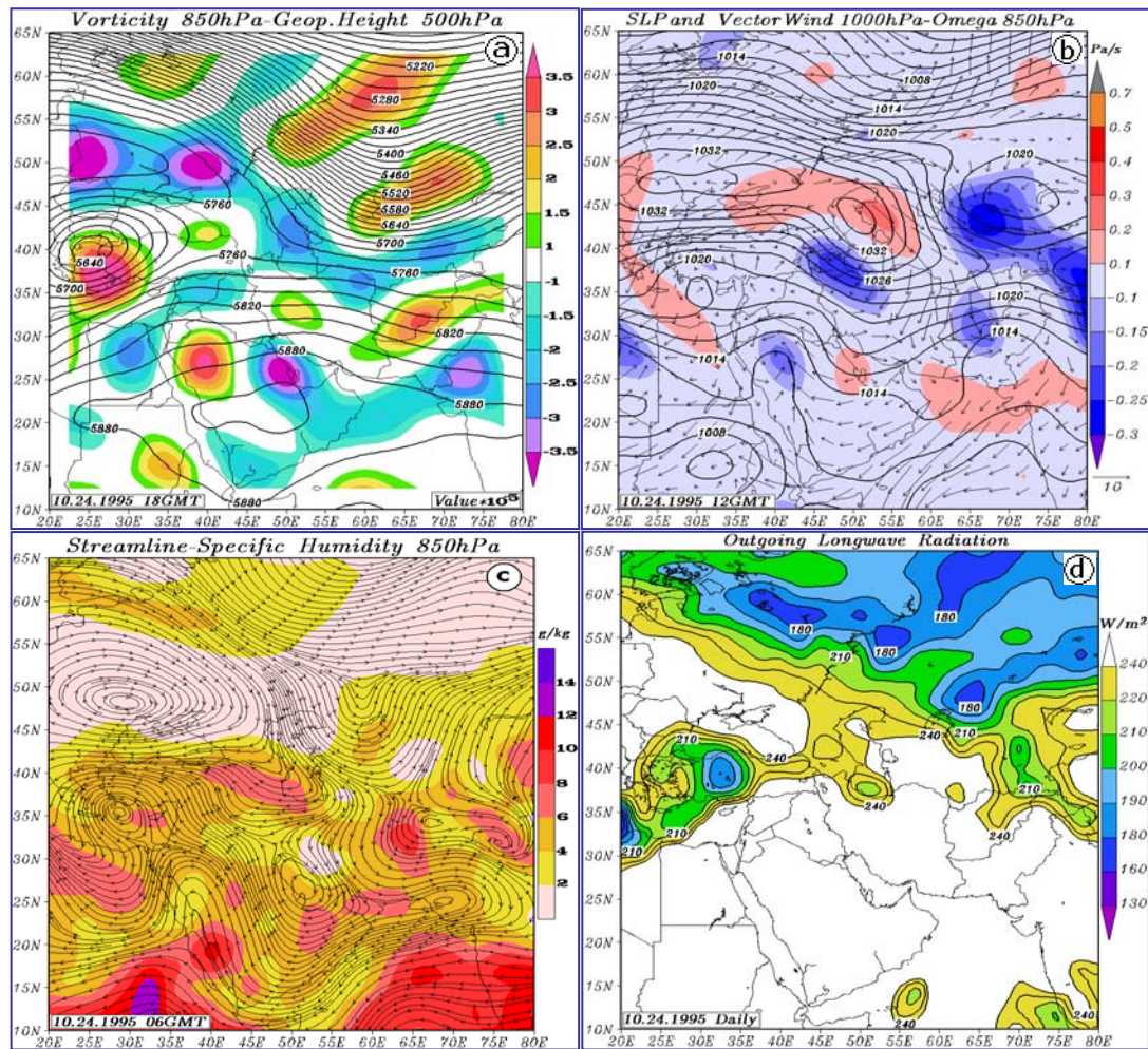
شکل ۳. نقشه‌های ترکیبی مربوط به الگوی پرفشار. الگوی نمونه مربوط به روز ۲۴ اکتبر ۱۹۹۵. (a) وضعیت همدیدی تراز ۵۰۰ هکتوپاسکال (gpm) و تاوایی نسبی ( 10^{-5} s^{-1} ) تراز ۸۵۰ هکتوپاسکال در ساعت ۱۸ گرینویچ. (b) فشار در سطح دریا-أمگا (Pa/s) در تراز ۸۵۰ هکتوپاسکال و بردار باد در تراز ۱۰۰۰ هکتوپاسکال در ساعت ۱۲ گرینویچ. (c) نم ویژه (g/kg) و خطوط جریان در تراز ۸۵۰ هکتوپاسکال در ساعت ۶ گرینویچ. (d) متوسط روزانه OLR ( W/m^2 ). در شکل‌ها از نشان تاوایی -۱ الی +۱ ( 10^{-5} s^{-1} ) و OLR کمتر از ۲۴۰ وات بر متر مربع صرف‌نظر شده است.
