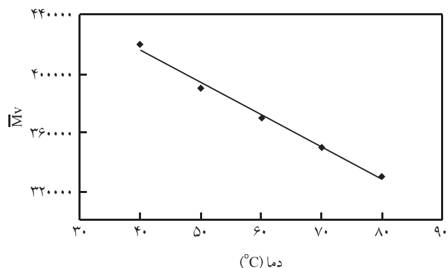
شکل ۶- اثر دمای کوپلیمر شدن بر وزن مولکولی متوسط گرانیوی پلیمر (\bar{M}_n) .
