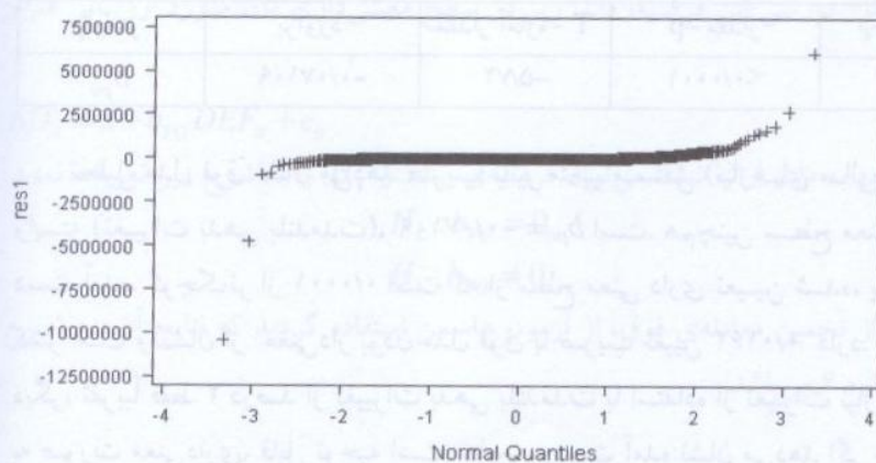
نمودار ۵: نرمال بودن باقی‌مانده‌های فرضیه‌ی دوم
