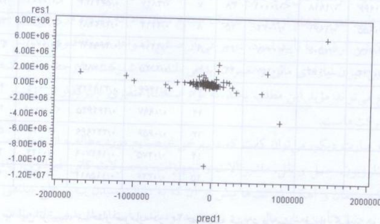
نمودار ۷: پراکنش مقادیر خطا فرضیه دوم
