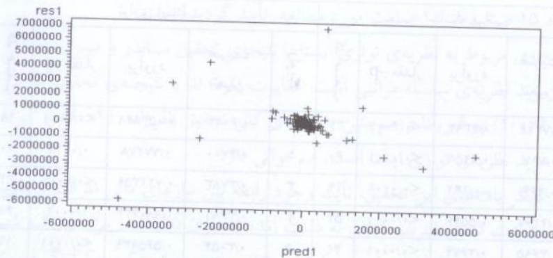
نمودار ۶: پراکنش مقادیر خطا فرضیه اول
