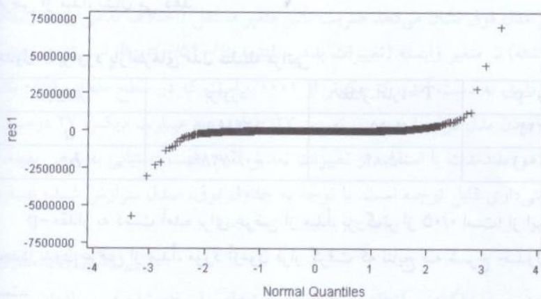
نمودار ۴: نرمال بودن باقی‌مانده‌های فرضیه‌ی اول
