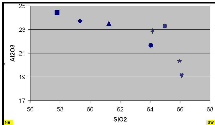
شکل ۵ تغییرات میزان آلومینا نسبت به میزان سیلیس.
