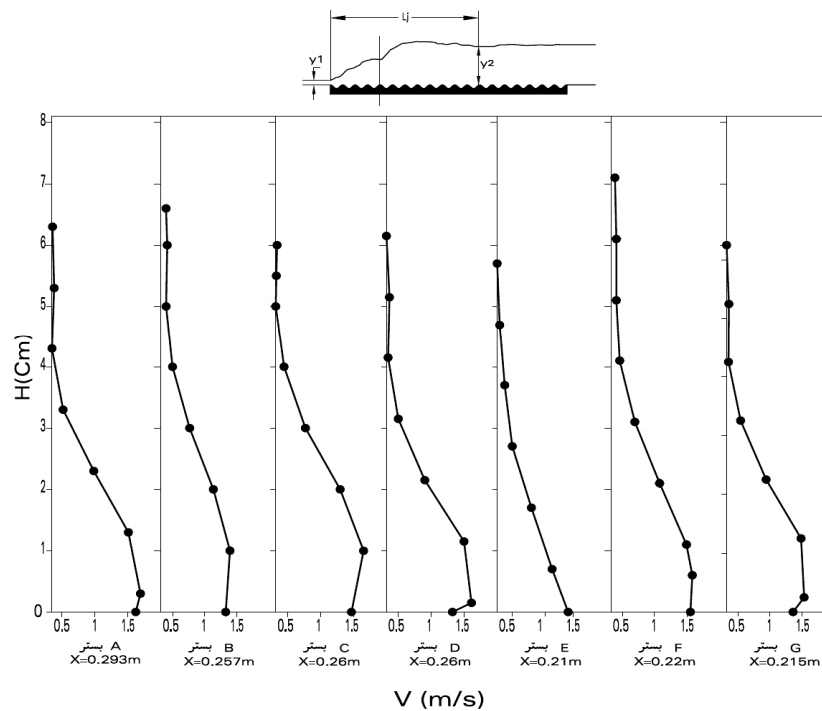
شکل ۱۰- پروفیل‌های سرعت روی بستر افقی موج‌دار در سه مقطع، یک سوم ابتدای پرش، یک سوم میانی و یک سوم انتهای پرش روی بسترهای موج‌دار سینوسی
