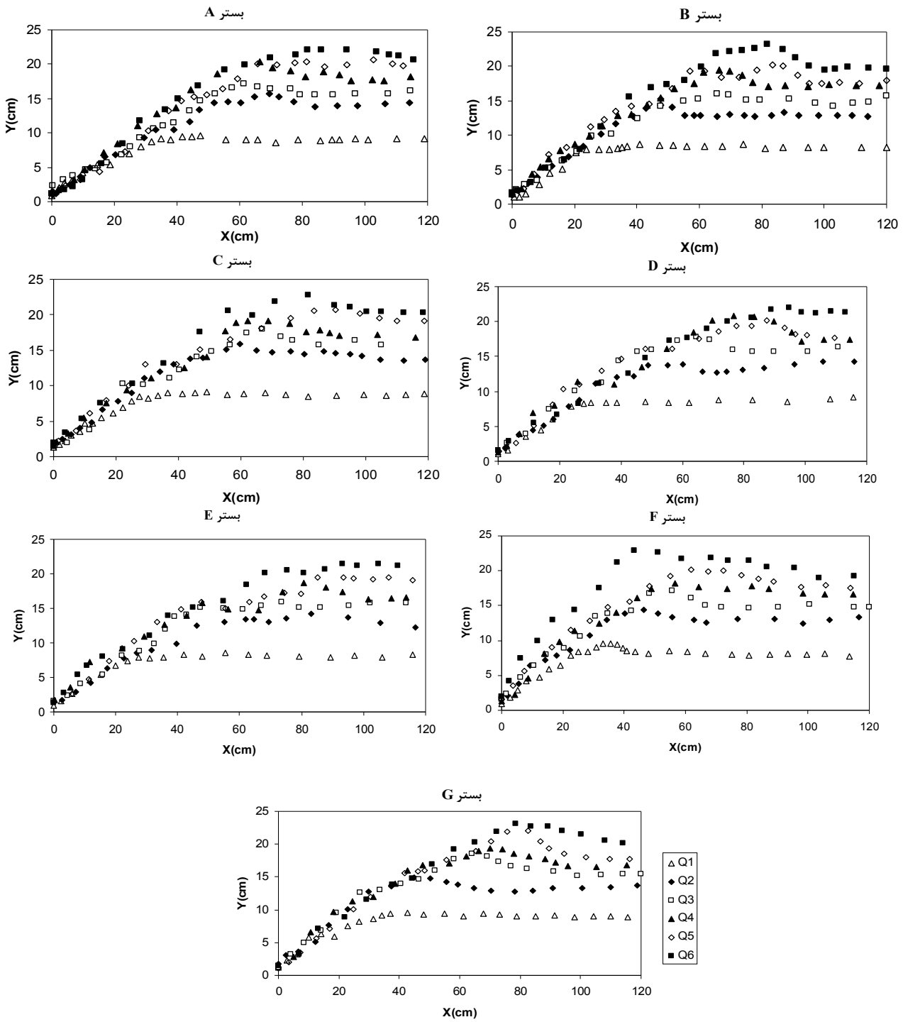
شکل ۲- پروفیل سطح آب در پخش هیدرولیکی
