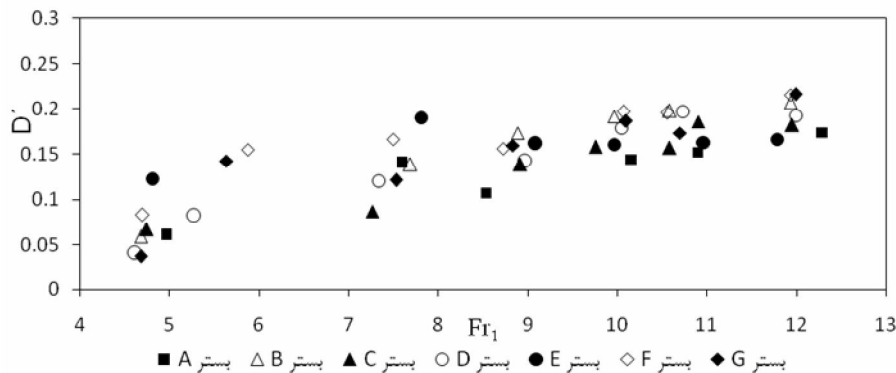
شکل ۵- تغییرات مقدار کاهش عمق نسبی پرش هیدرولیکی نسبت به اعداد فرود اولیه
