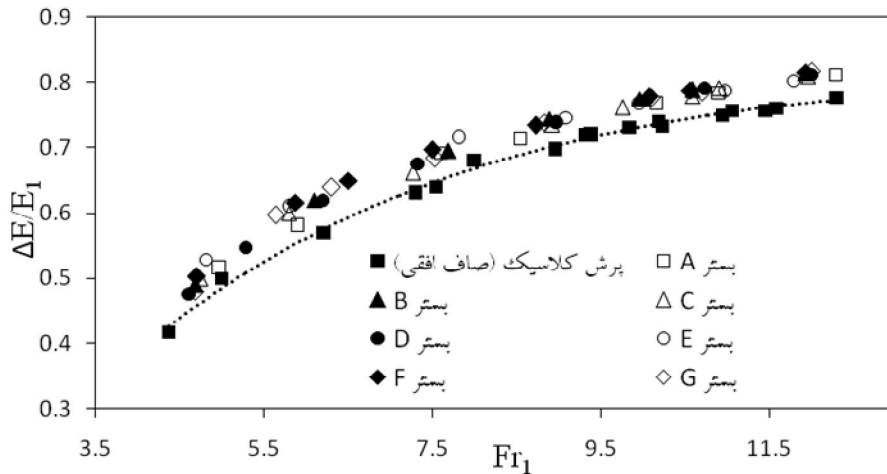
شکل ۷- تغییرات اتلاف انرژی نسبی پرش روی بسترهای موج‌دار سینوسی و صاف به ازای اعداد فرود اولیه
