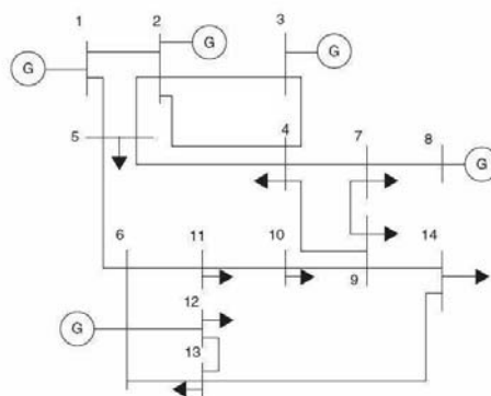
شکل (۴): شبکه ۱۴ باسه استاندارد IEEE
