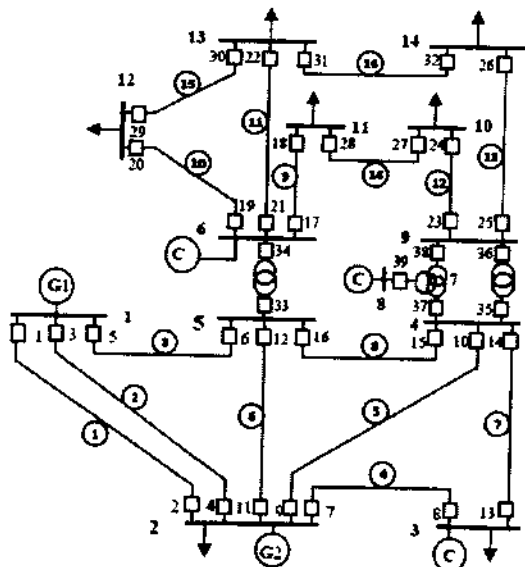
شکل (۲): دیاگرام تک خطی شبکه ۱۴ شینه IEEE
