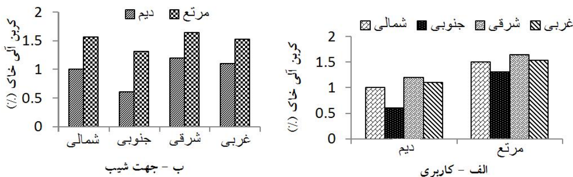
نمودار ۱- تاثیر کاربری و جهت گوناگون شیب بر میزان کربن آلی خاک
