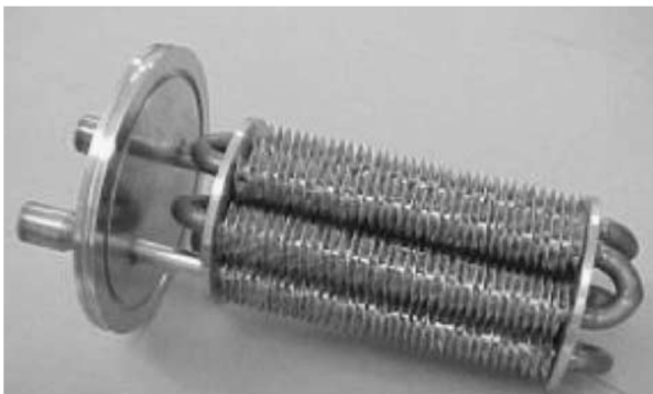
شکل ۲ بسترهای ماده جذب با فین‌های حلقوی که داخل محفظه قرار می‌گیرند
