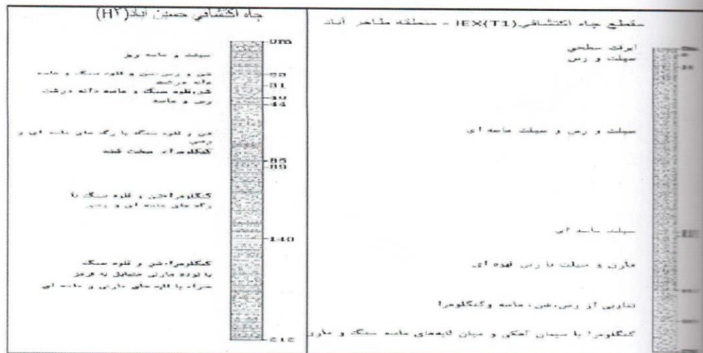
شکل (۵): نمونه ای از لاگ چاه‌های اکتشافی در حسین آباد و طاهر آباد.
