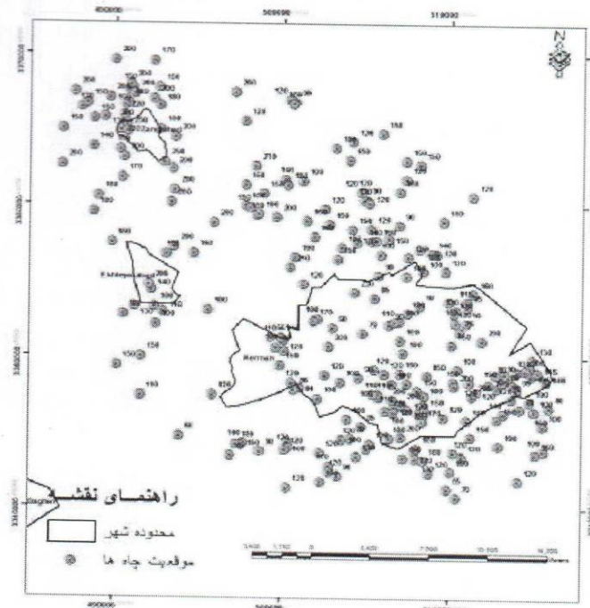
شکل (۸): نقشه پراکنش چاه‌های بهره‌برداری و پیزومتری دشت کرمان
