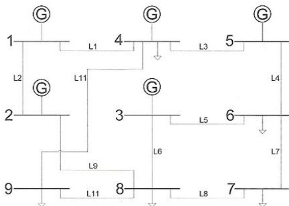
شکل ۱: دیاگرام شبکه ۹ باسه اصلاح شده.
