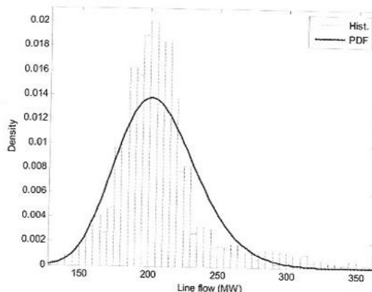
شکل ۴: منحنی فراوانی و تابع چگالی احتمال توان جاری خط ۹.
