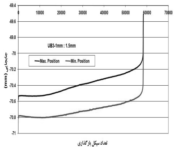
شکل ۲۵ نمودار جابه جایی - تعداد دوره بارگذاری برای نمونه ۱۵-۱۰-UB، P_{max}=500N (شروع انتشار ترک تقریباً در ۱۲۰۰۰ سیکل)
