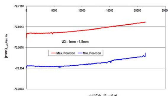
شکل ۲۰ نمودار جابه‌جایی - تعداد دوره بارگذاری برای نمونه UA۱۰-۱۵-۳، P_{max}=350N (شروع انتشار ترک تقریباً در ۶۰۰۰ سیکل)
