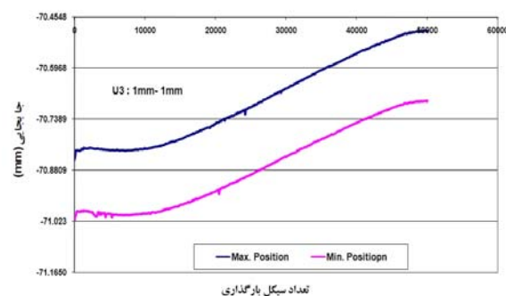
شکل ۱۹ نمودار جابه‌جایی - تعداد دوره بارگذاری برای نمونه UA۱۰-۱۰-۳، P_{max}=350N (شروع انتشار ترک تقریباً در ۹۰۰۰ سیکل)
