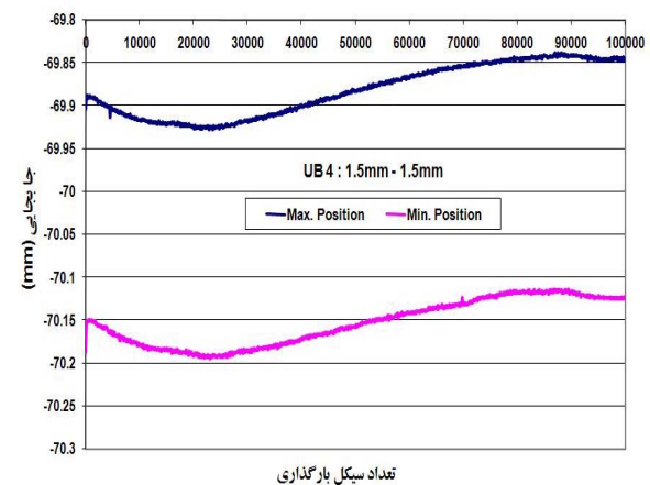
شکل ۲۶ نمودار جابه جایی - تعداد دوره بارگذاری برای نمونه ۱۵-۱۵-UB، P_{max}=900N (شروع انتشار ترک تقریباً در ۲۵۰۰۰ سیکل)
