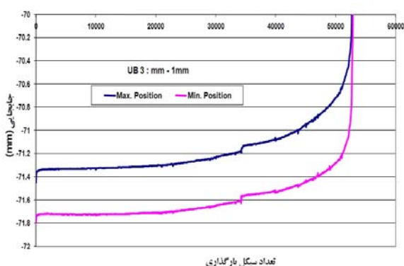
شکل ۲۴ نمودار جابه‌جایی - تعداد دوره بارگذاری برای نمونه UB۱۰-۱۰-۳، P_{max}=500N (شروع انتشار ترک تقریباً در ۱۲۰۰۰ سیکل)
