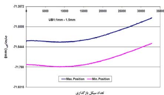
شکل ۲۲ نمودار جابه‌جایی - تعداد دوره بارگذاری برای نمونه UB۱۰-۱۵-۱، P_{max}=350N (شروع انتشار ترک تقریباً در ۱۲۵۰۰ سیکل)
