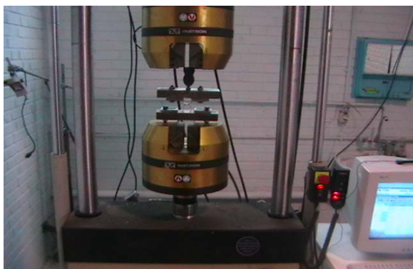
شکل ۲ نحوه قرار گرفتن نمونه‌ها در دستگاه تست خستگی
