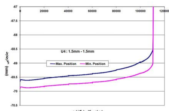
شکل ۲۱ نمودار جابه‌جایی - تعداد دوره بارگذاری برای نمونه UA۱۵-۱۵-۴، P_{max}=900N (شروع انتشار ترک تقریباً در ۱۵۰۰۰ سیکل)
