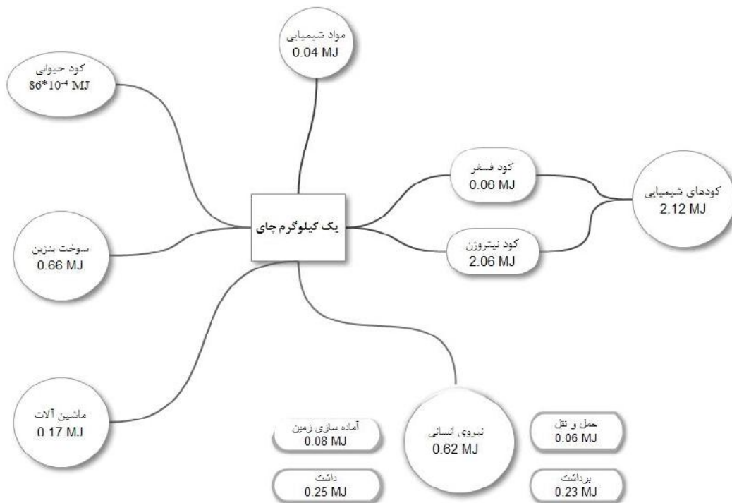
شکل ۲. جریان انرژی تولید یک کیلوگرم چای در استان گیلان
