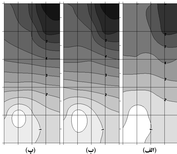
شکل ۲- کنتور اختلاف اندیس نشت بین تحلیل های همزمان و مجزا
