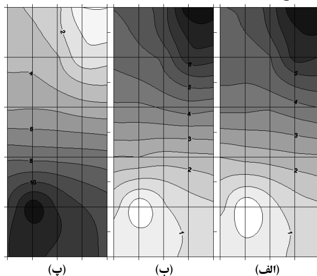
شکل ۴- بررسی محل کمترین اختلاف بین جواب تحلیل های مجزا و همزمان الف) Q_{i^{19}} = 20 \text{ l/s} و Q_{i^{11}} = 20 \text{ l/s} (ب) Q_{i^{19}} = 20 \text{ l/s} و Q_{i^{11}} = 50 \text{ l/s} (پ) Q_{i^{19}} = 20 \text{ l/s} و Q_{i^{11}} = 5 \text{ l/s}
