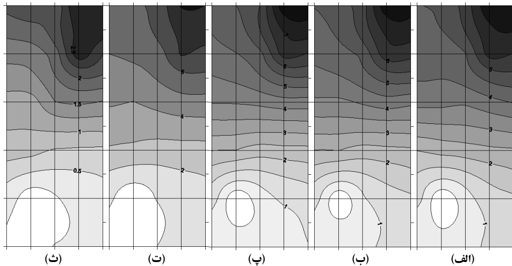
شکل ۳- کنتور اختلاف اندیس نشت بین تحلیل های همزمان و مجزا با دبی پایه ۵۰ لیتر بر ثانیه الف) Q_{i^{19}} = 20 \text{ l/s} و Q_{i^{11}} = 20 \text{ l/s} (ب) Q_{i^{19}} = 20 \text{ l/s} و Q_{i^{11}} = 50 \text{ l/s} (پ) Q_{i^{19}} = 20 \text{ l/s} و Q_{i^{11}} = 100 \text{ l/s} (ت) Q_{i^{19}} = 5 \text{ l/s} و Q_{i^{11}} = 20 \text{ l/s} (ث) Q_{i^{19}} = 1 \text{ l/s} و Q_{i^{11}} = 20 \text{ l/s}
