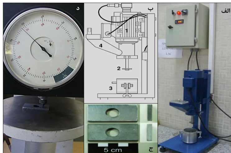
شکل ۱. الف) دستگاه سایش LCPC (دانشگاه فردوسی مشهد)، ب) شکل شماتیک دستگاه LCPC (۱) موتور، ۲) ایملر، ۳) ظرف نمونه، ۴) فانل تیوب (Funnel Tube)، ج) نمونه ایملر و د) اندازه‌گیری سختی راکول (HRB ۶۸)
