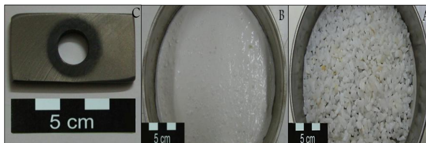
شکل ۲. A و B) نمونه کوارتز قبل و پس از آزمایش LCPC (آزمایش تأثیر آب)، C) ایملر استفاده شده پس از آزمایش
