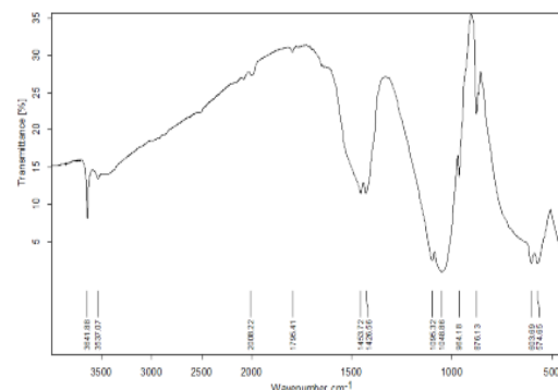
شکل ۴: طیف FTIR نمونه پودری FAp-10wt.% TiO 2 پس از عملیات حرارتی در دمای ۵۵۰ °C.
