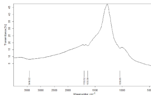
شکل ۳: طیف FTIR نمونه پودری TiO 2 پس از عملیات حرارتی در دمای ۵۵۰ °C.
