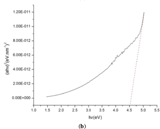
شکل ۷: (a) منحنی جذب اشعه UV و (b) منحنی Tauc نمونه فلئورآپاتیت خالص.
