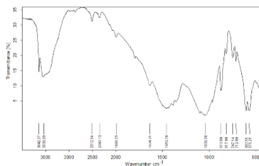
شکل ۲: طیف FTIR نمونه پودری FAp پس از عملیات حرارتی در دمای ۵۵۰ °C.
