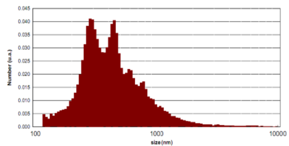
شکل ۵: توزیع اندازه ذرات برای نمونه FAp.
