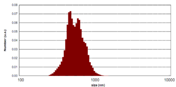
شکل ۶: توزیع اندازه ذرات برای نمونه FAp-TiO 2 .
