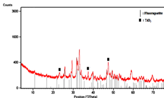
شکل ۱: طیف XRD نمونه فلوئورآپاتیت/تیتانیا حاوی ۱۰٪ وزنی تیتانیا پس از عملیات حرارتی در دمای ۵۵۰ °C.
