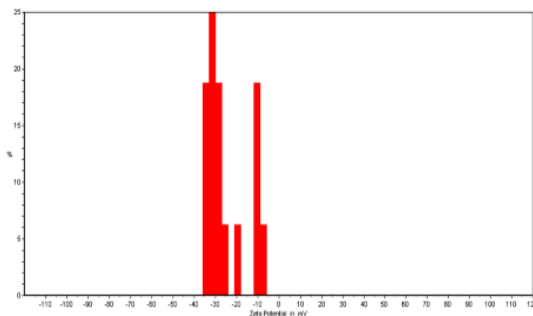
شکل ۱۲: توزیع مقادیر پتانسیل زتا برای نمونه \text{FAP-10wt.\%TiO}_2 در محلول SBF و در دمای ۳۷ درجه سانتیگراد.
