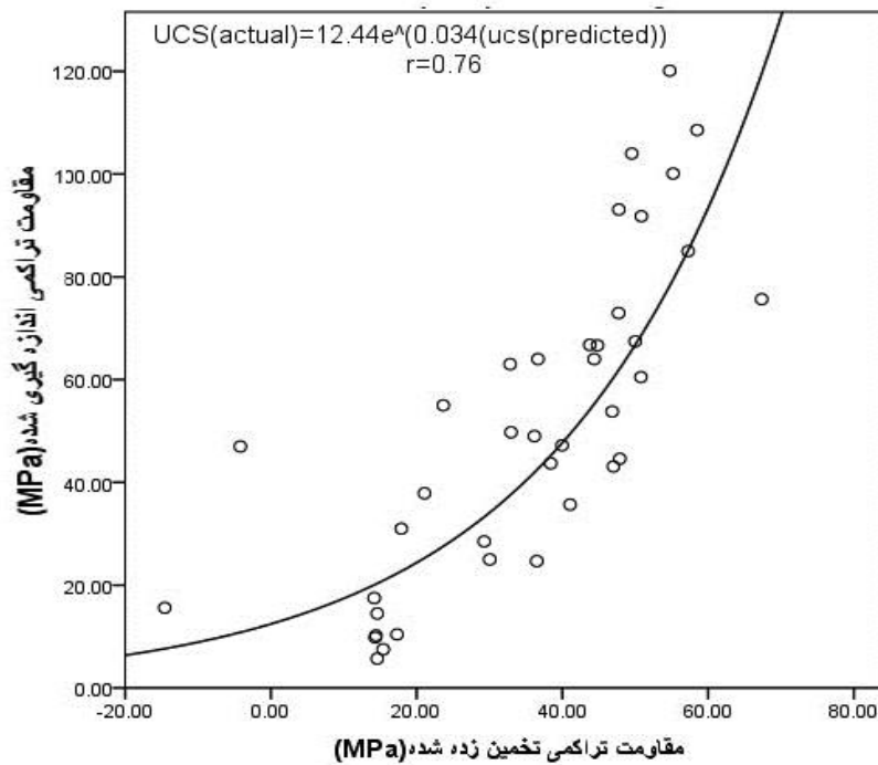
شکل 7. رابطه بین مقاومت تراکمی تک‌محوری تخمین زده شده توسط رابطه‌ی ۳ با مقادیر مقاومت تراکمی تک‌محوری اندازه‌گیری شده
