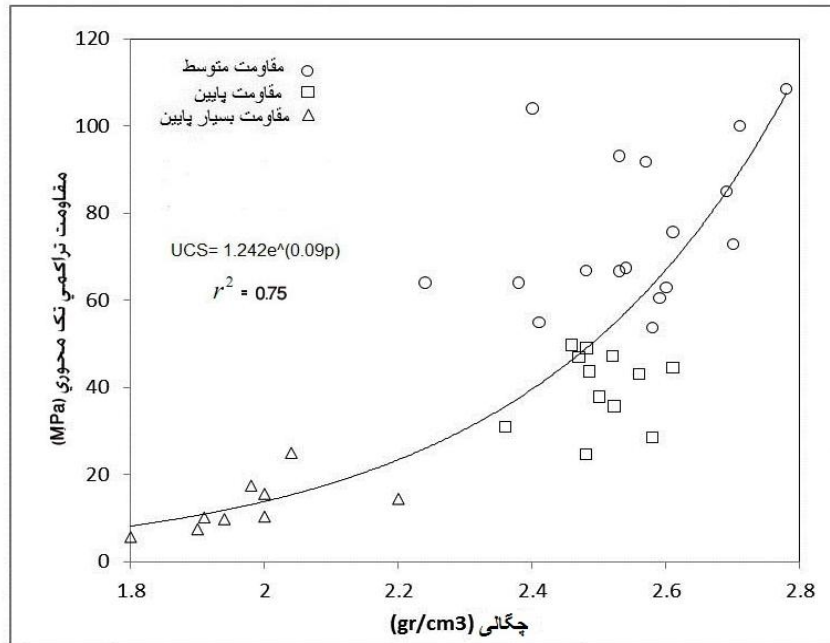
شکل 4. رابطه‌ی چگالی در مقابل مقاومت تراکمی تک محوری
