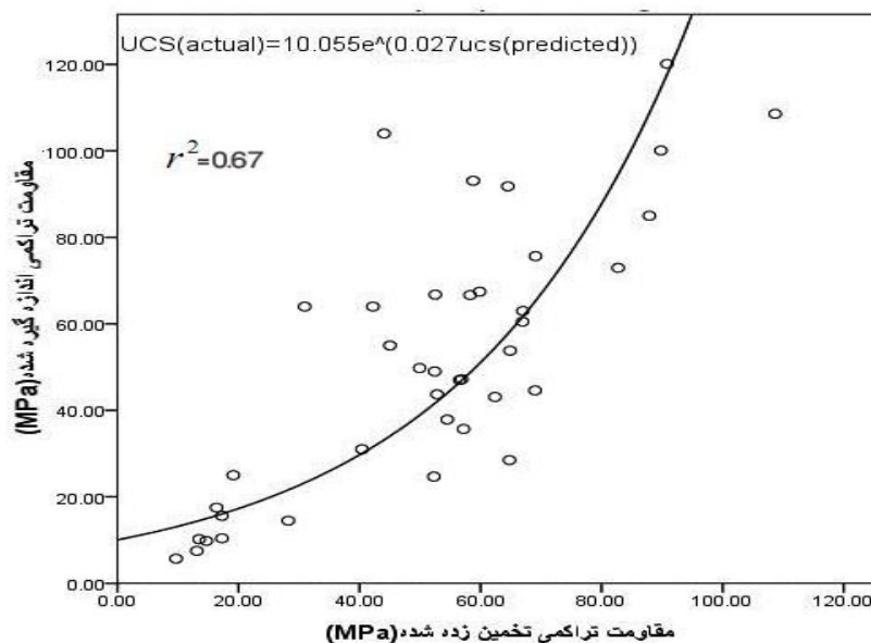
شکل 5. رابطه بین مقاومت تراکمی تک محوری تخمین زده شده توسط رابطه‌ی 1 با مقادیر مقاومت تراکمی تک محوری اندازه گیری شده
