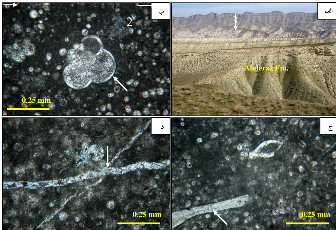
شکل 2- الف) سازند آبدراز در ناحیه مورد مطالعه که از شیل و مارن‌های خاکستری و سنگ‌های گل‌سفیدی تشکیل شده است. ب) مقطع میکروسکوپی از سنگ آهک‌های گل‌سفیدی متشکل از روزن‌داران. ج) خرده دوکفه‌ای در سنگ آهک گل‌سفیدی. د) رگه‌های متقاطع پر شده توسط کلسیت اسپاری در سنگ آهک‌های گل‌سفیدی منطقه.
