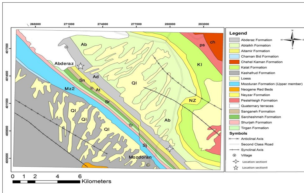
شکل 1. محدوده مورد مطالعه برگرفته شده از نقشه زمین‌شناسی 1/250000 سرخس (Afshar-Harb, 1982)
