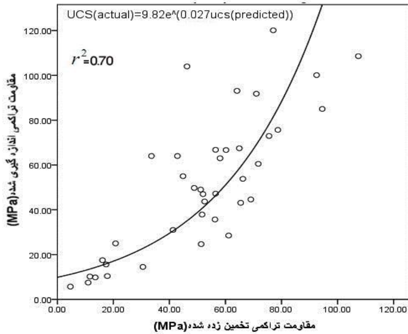
شکل 6. رابطه بین مقاومت تراکمی تک‌محوری تخمین زده شده توسط رابطه‌ی ۲ با مقادیر مقاومت تراکمی تک‌محوری اندازه‌گیری شده
