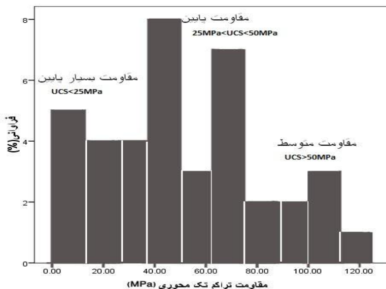
شکل 3. نمودار توزیع تجمعی مقاومت تراکمی تک‌محوری
