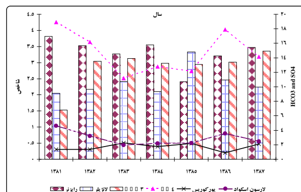
شکل ۶- روند تغییرات شاخص‌های خوردگی و رسوب‌گذاری در مقابل تغییرات SO_4 و HCO_3
