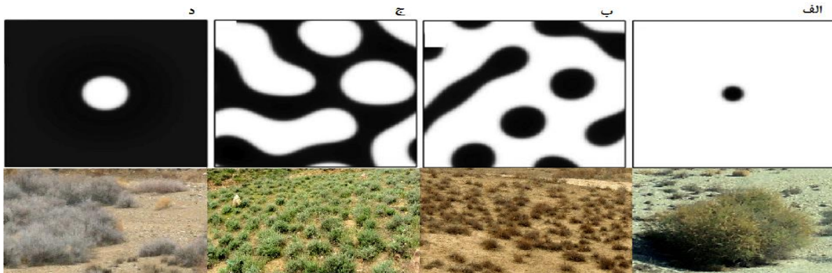
شکل ۵. الگوهای ترکیبی در محدوده‌های پایداری دوجانبه بر اساس مدل جیلاد و تطابق آن با الگوهای موجود در اکوسیستم‌های خشک ایران (الف) وضعیت فاقد پوشش همراه الگوی نقطه‌ای، (ب) الگوی نقطه‌ای و خطی، (ج) خطی و درزی، (د) الگوی درزی و وضعیت همگن پوششی. نقاط تیره بیانگر تراکم بایومس است (نویسندگان اثر این تصاویر را در سال ۱۳۹۲ از اکوسیستم‌های خراسان رضوی تهیه کرده‌اند).
