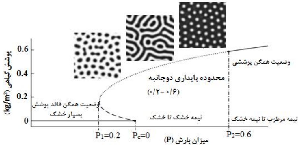
شکل ۴. دیاگرام انشعاب برای وضعیت‌های همگن پوششی و فاقد پوشش در امتداد شیب بارش بر اساس مدل جیلاد
