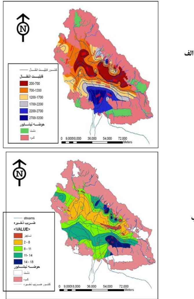
شکل ۴- الف) نقشه هم مقدار قابلیت انتقال (متر مربع بر روز) در محدوده دشت نیشابو ب) ضریب ذخیره آبخوان در مهر ۱۳۸۵ در محدوده دشت نیشابو
