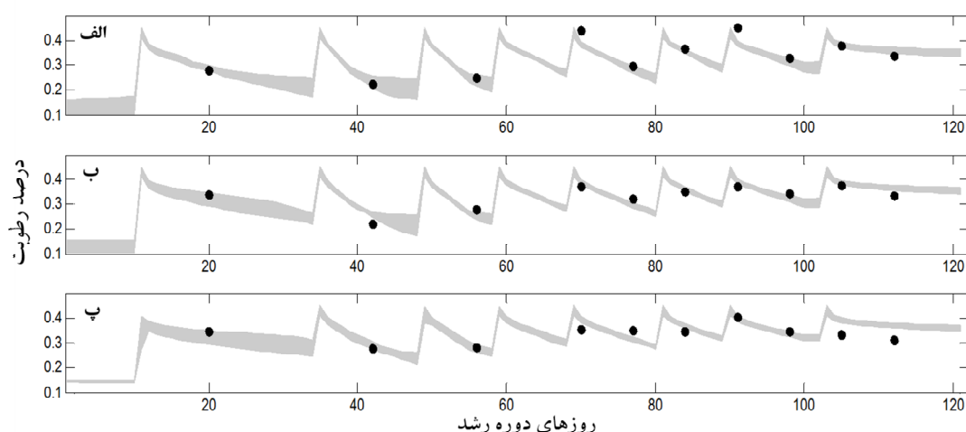
شکل ۳- بازه اطمینان ۹۵٪ رطوبت پیش‌بینی شده (بخش سایه‌خورده) و مقادیر اندازه‌گیری شده (نقاط) آن (در عمق‌های الف: ۱۵-، ب: ۳۰-۱۵ و پ: ۶۰-۳۰ سانتی‌متر)
