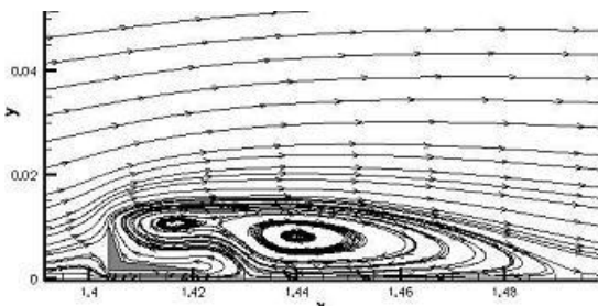
شکل ۷- خطوط جریان حول گونیا (برگرفته از مرجع [۱])
