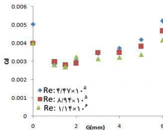
شکل ۶- ضریب پسای متوسط صفحه‌ی تخت بر حسب فاصله‌ی گونیا از صفحه در رینولدزهای مختلف
