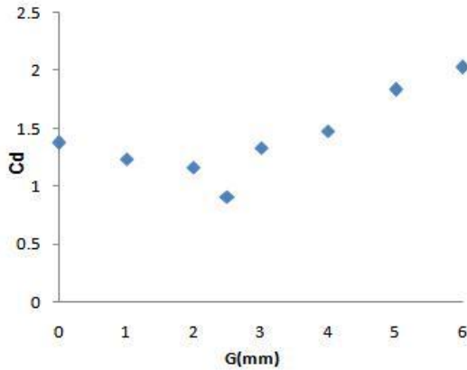
شکل ۳- ضریب پسای متوسط مانع مربعی بازای فواصل مختلف مانع از صفحه در عدد رینولدز 8.94 \times 10^5
