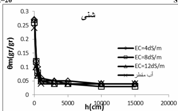
شکل ۳- منحنی مشخصه رطوبتی در شوری‌های متفاوت و در SAR=20
