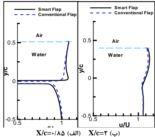
شکل ۱۳- پروفیل سرعت (الف) در ناحیه وسط بالچه، (ب) پشت هیدروفویل در شرایط AOF = -7.5^\circ و h/c = 0.5
