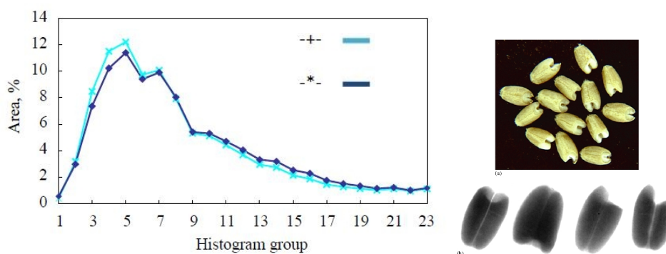
شکل ۷ - تصویر سمت راست نمونه ناسالم از گندم با تصویر x-ray و سمت چپ مربوط به هیستوگرام دانه های ناسالم -+ و سالم -*
