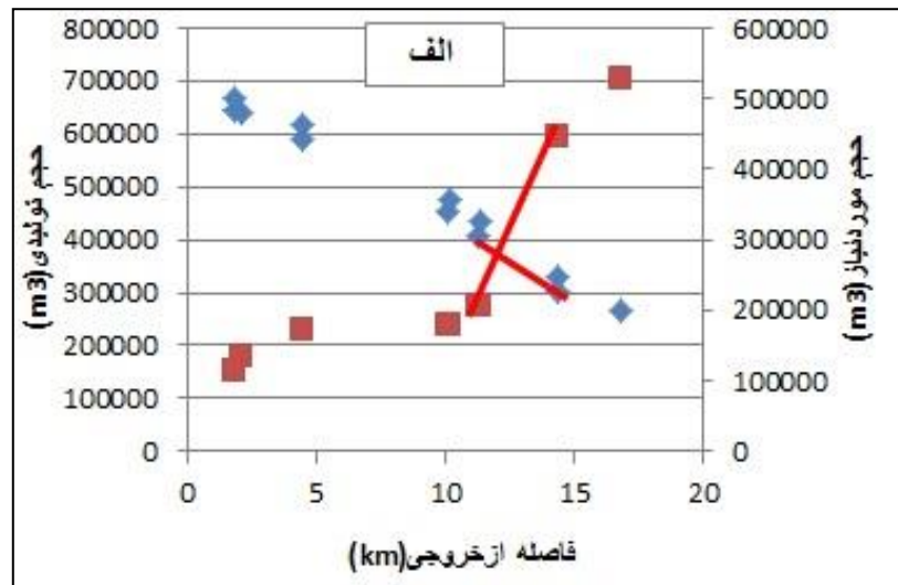
ادامه شکل ۳: مقایسه حجم آب مورد نیاز اراضی پایین دست با رواناب تولیدی در بالادست برای الف: انشعاب راست آبراهه ب: انشعاب چپ آبراهه (اشکال مربع نماینده حجم آب مورد نیاز و اشکال لوزی نماینده حجم رواناب تولیدی هستند)
