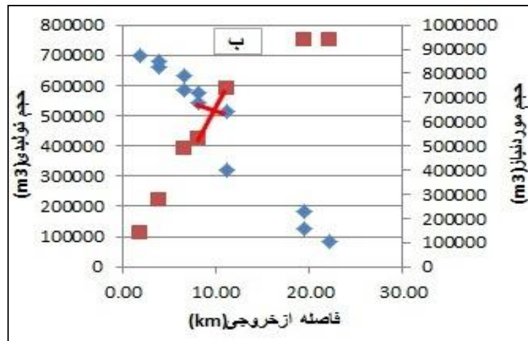
شکل ۳: مقایسه حجم آب مورد نیاز اراضی پایین دست با رواناب تولیدی در بالادست برای الف: انشعاب راست آبراهه ب: انشعاب چپ آبراهه (اشکال مربع نماینده حجم آب مورد نیاز و اشکال لوزی نماینده حجم رواناب تولیدی هستند)
