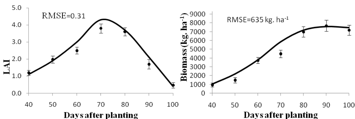
شکل ۱- مقادیر شبیه‌سازی شده (خطوط) و مشاهده شده (نقاط) شاخص سطح برگ و ماده خشک تولیدی نخود در مشهد Fig. 1- Comparison of simulated (lines) and observed (data points) values of leaf area index (LAI) and above ground biomass of chickpea in Mashhad
