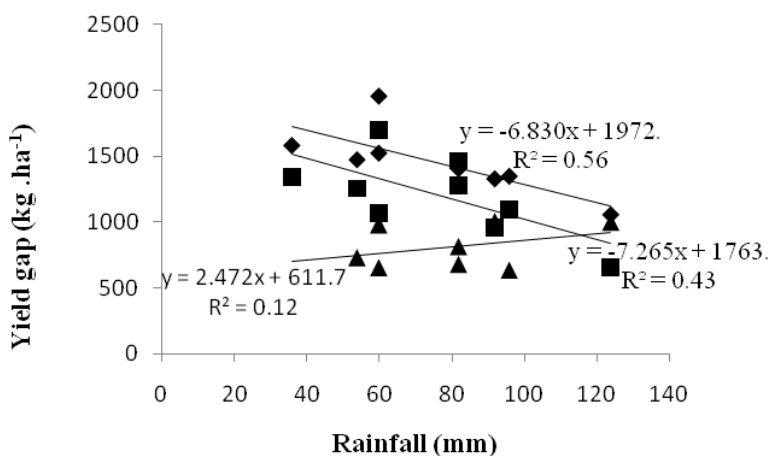
شکل ۶- رابطه خلاء بین عملکرد پتانسیل آبی و عملکرد واقعی آبی (♦)، خلاء بین عملکرد پتانسیل آبی و دیم شبیه‌سازی (■) و خلاء بین عملکرد پتانسیل دیم و عملکرد واقعی دیم (▲) با بارندگی طی دوران رشد در مناطق مورد مطالعه در استان خراسان رضوی.
