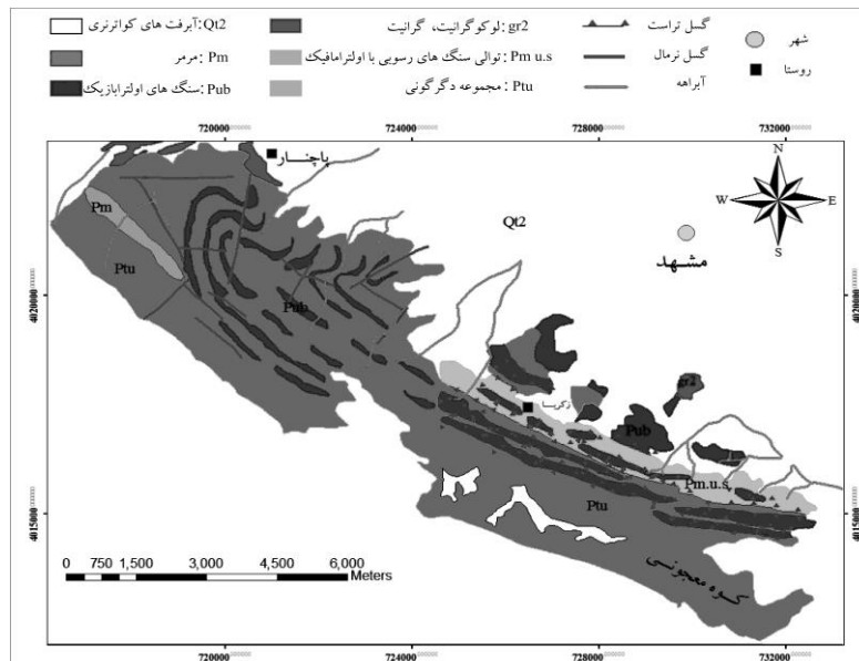
شکل ۳. نقشه زمین‌شناسی رقومی شده منطقه مورد مطالعه (برگرفته از نقشه ۱:۱۰۰۰۰۰ مشهد و طبقه)
