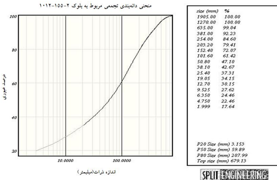
شکل ۸. منحنی توزیع دانه بندی بدست آمده برای یک کپه انفجاری
