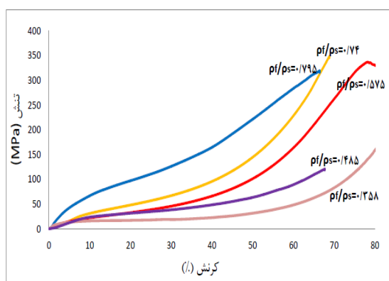
شکل (۱۰): نتایج آزمون فشار فوم‌های تولیدشده با ۲ درصد وزنی نانو ذرات آلومینا و درصد‌های تخلخل متفاوت
