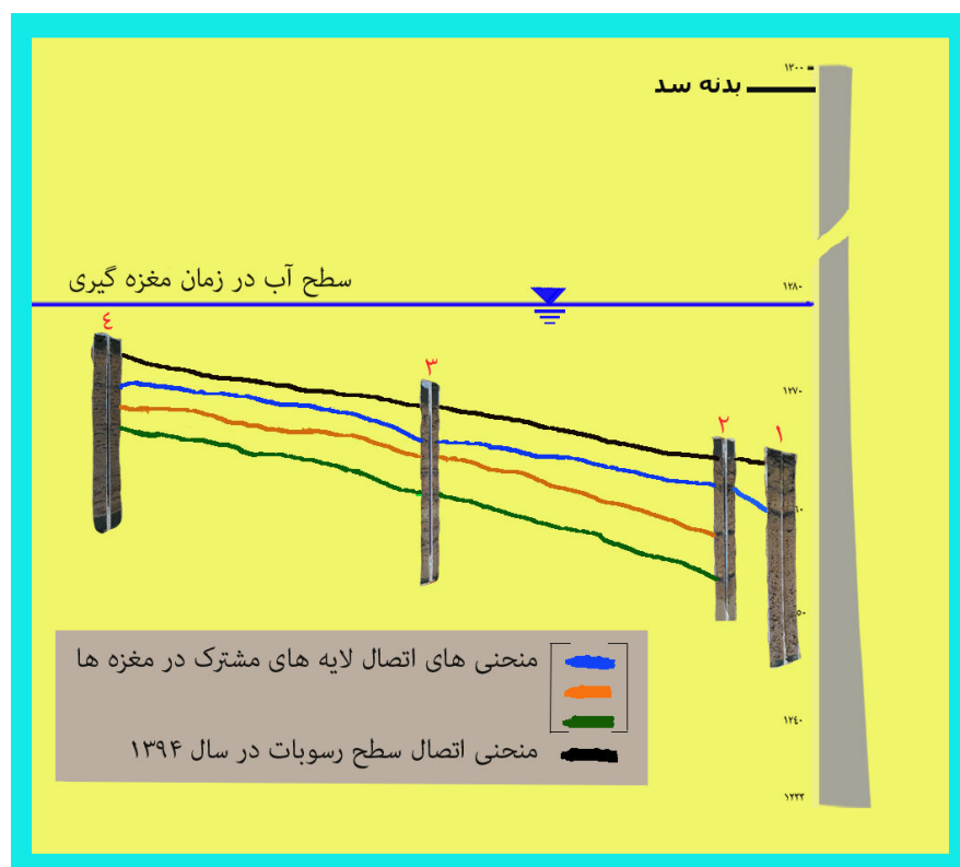
شکل ۵- تصویری شماتیک از پروفیل مخزن
