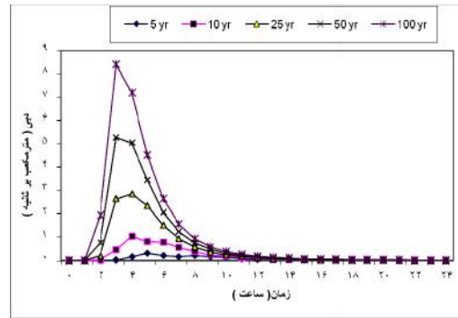
شکل ۱۶- آنمود سیل در زمان قبل از اقدامات آبخیزداری.
