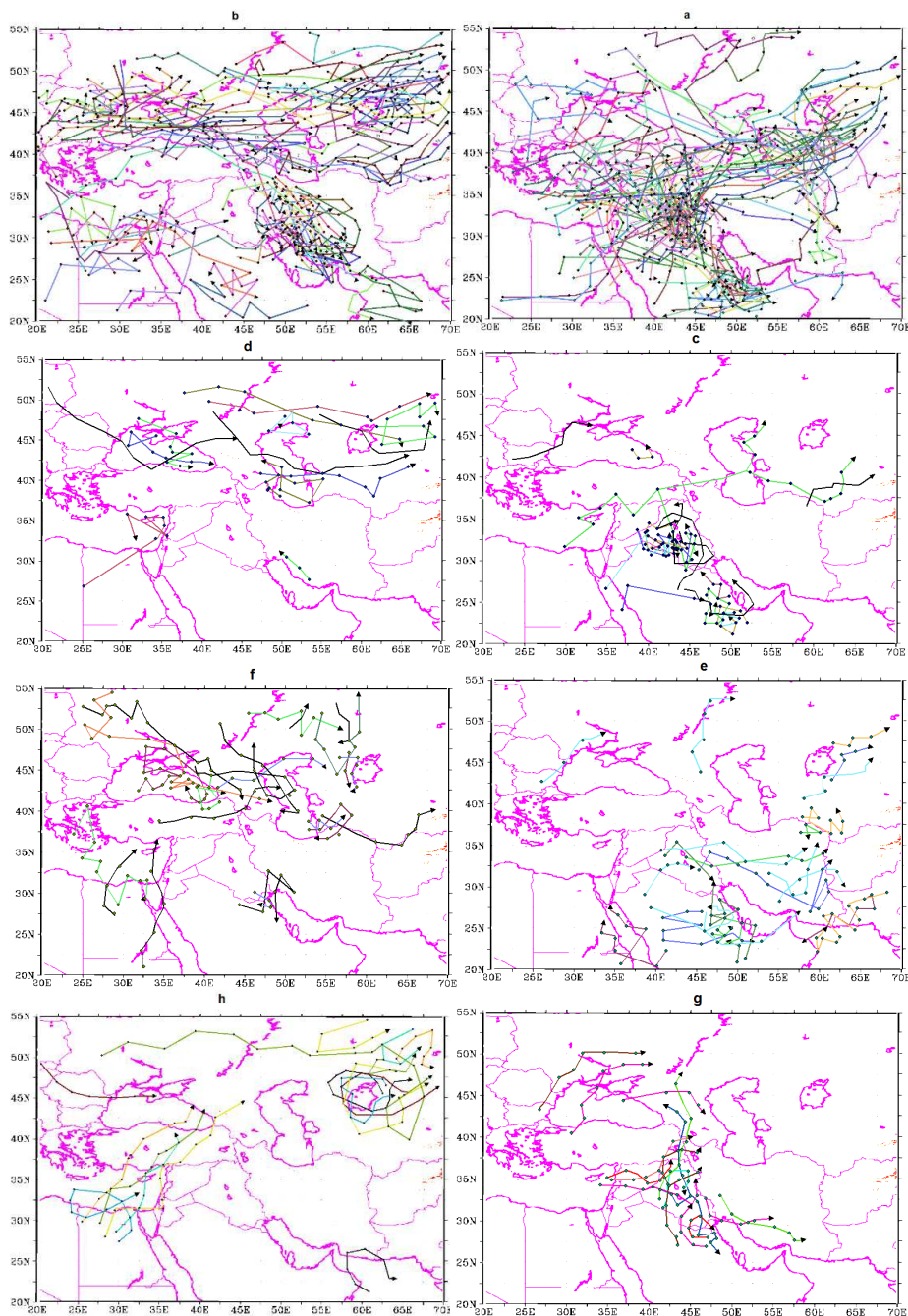
شکل ۱۱: تعیین موقعیت و مسیر جابجایی ۶ ساعته چرخندها و واچرخندهای مهاجر و فعال به تفکیک برای روزهای متعلق به چهار الگوی همدیدی. (a) چرخندهای مربوط به الگوی اول (b) واچرخندهای مربوط به الگوی اول (c) چرخندهای مربوط به الگوی دوم (d) واچرخندهای مربوط به الگوی دوم (e) چرخندهای مربوط به الگوی سوم (f) واچرخندهای مربوط به الگوی سوم (g) چرخندهای مربوط به الگوی چهارم (h) واچرخندهای مربوط به الگوی چهارم. (خطوط هم‌رنگ، مسیر جابجایی چرخندها و واچرخندها فعال در هر روز را نمایش می‌دهد).
