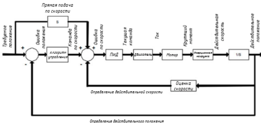
Рис. 2. Структурная схема feed-forward регулятора
