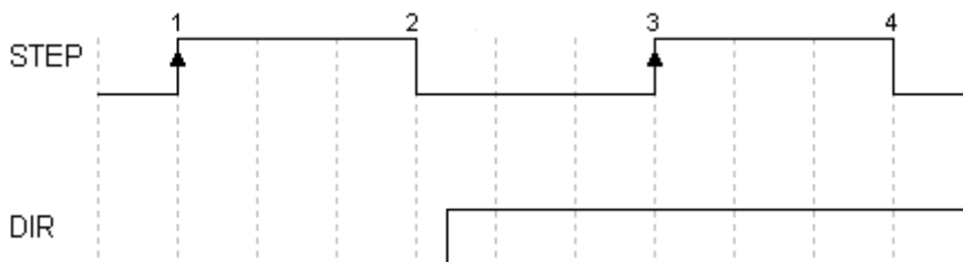
Рис. 3. Вид управляющего сигнала протокола step/dir
