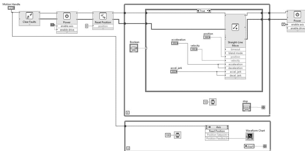
Рис. 5. Реализация системы управления прецизионным станком в формате графического языка G в среде разработки LabVIEW
