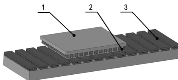
Рис. 2. Принципиальная схема линейного сервопривода: 1 – якорь; 2 – неподвижная часть; 3 – постоянные магниты
