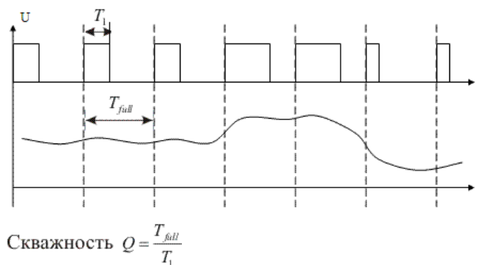
Рис. 4. Преобразование ШИМ сигнала в аналоговый \pm 10 В, видны колебания выходного управляющего сигнала
