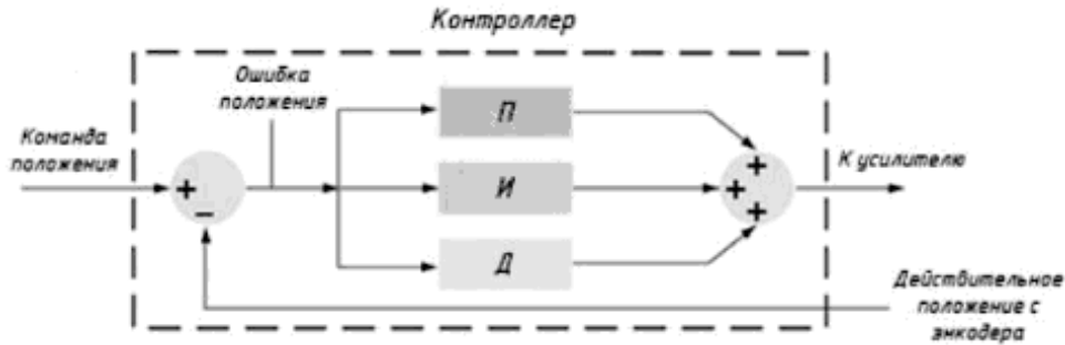
Рис. 1. Структурная схема ПИД-регулятора
