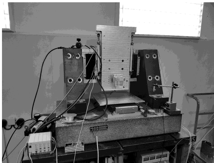
Рис. 1. Макет технологического оборудования – прецизионный фрезерный станок
