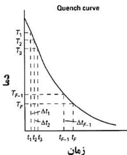
شکل ۳- منحنی سردشدن و طرح‌واره نمودار زمان-دما-خواص ( TTP ) رسم شده با استفاده از ثوابت روش محاسبه عامل کوینچ
