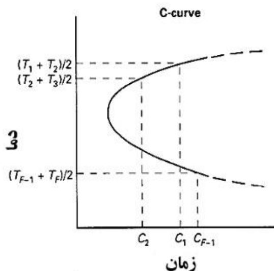
شکل ۳- منحنی سردشدن و طرح‌واره نمودار زمان-دما-خواص ( TTP ) رسم شده با استفاده از ثوابت روش محاسبه عامل کوینچ
