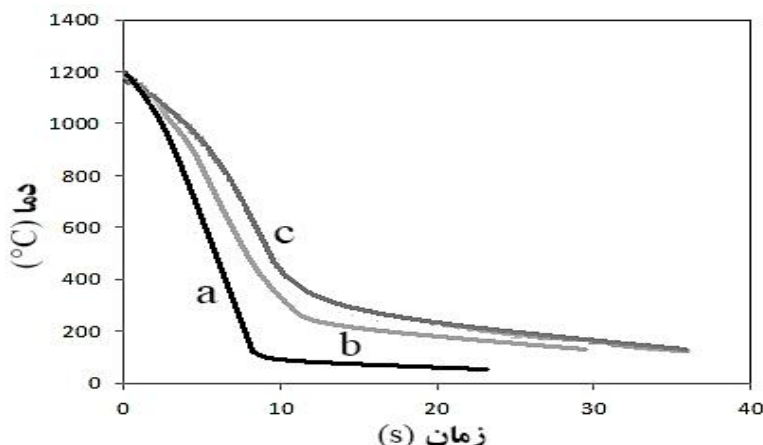
شکل ۴- منحنی‌های سردشدن نوعی در محیط‌های مختلف: (a)، محیط پلیمری 10^{\circ}\text{C} ، (b) روغن 50^{\circ}\text{C} ، (c) روغن 22^{\circ}\text{C}
