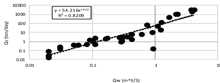
شکل ۲- منحنی سنجه رسوب زیر مدل ماه‌های فاقد پوشش گیاهی از مدل پوشش گیاهی در ایستگاه هیدرومتری گلستان جاغرغ Figure 2. Sediment Rating Curve for "sub-model of months without of vegetation" from the vegetations model in hydrometric station of Golestan Jagharq
