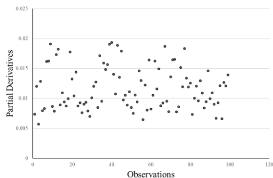
(خ) مشتق جزئی خروجی شبکه نسبت به نحوه خرید (خرده‌فروش) (i) The partial derivatives of network output with respect to type of purchase (buy from retailers).
