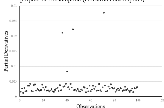
(ز) مشتق جزئی خروجی شبکه نسبت به بسته‌بندی (n) The partial derivatives of network output with respect to packing.
