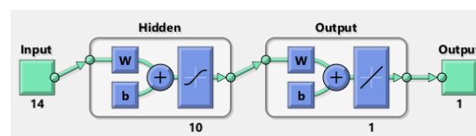
شکل ۱- ساختار شبکه عصبی مصنوعی طراحی شده
